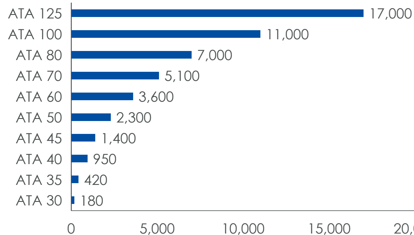
Maximum torque(N.m)
