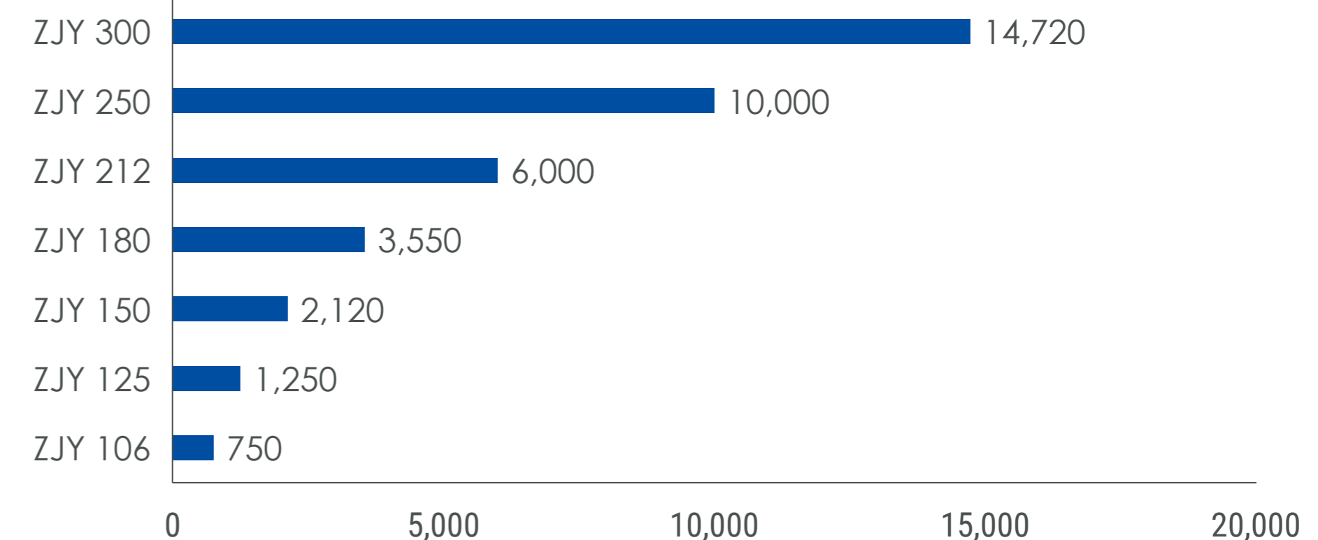
Maximum torque(N.m)
