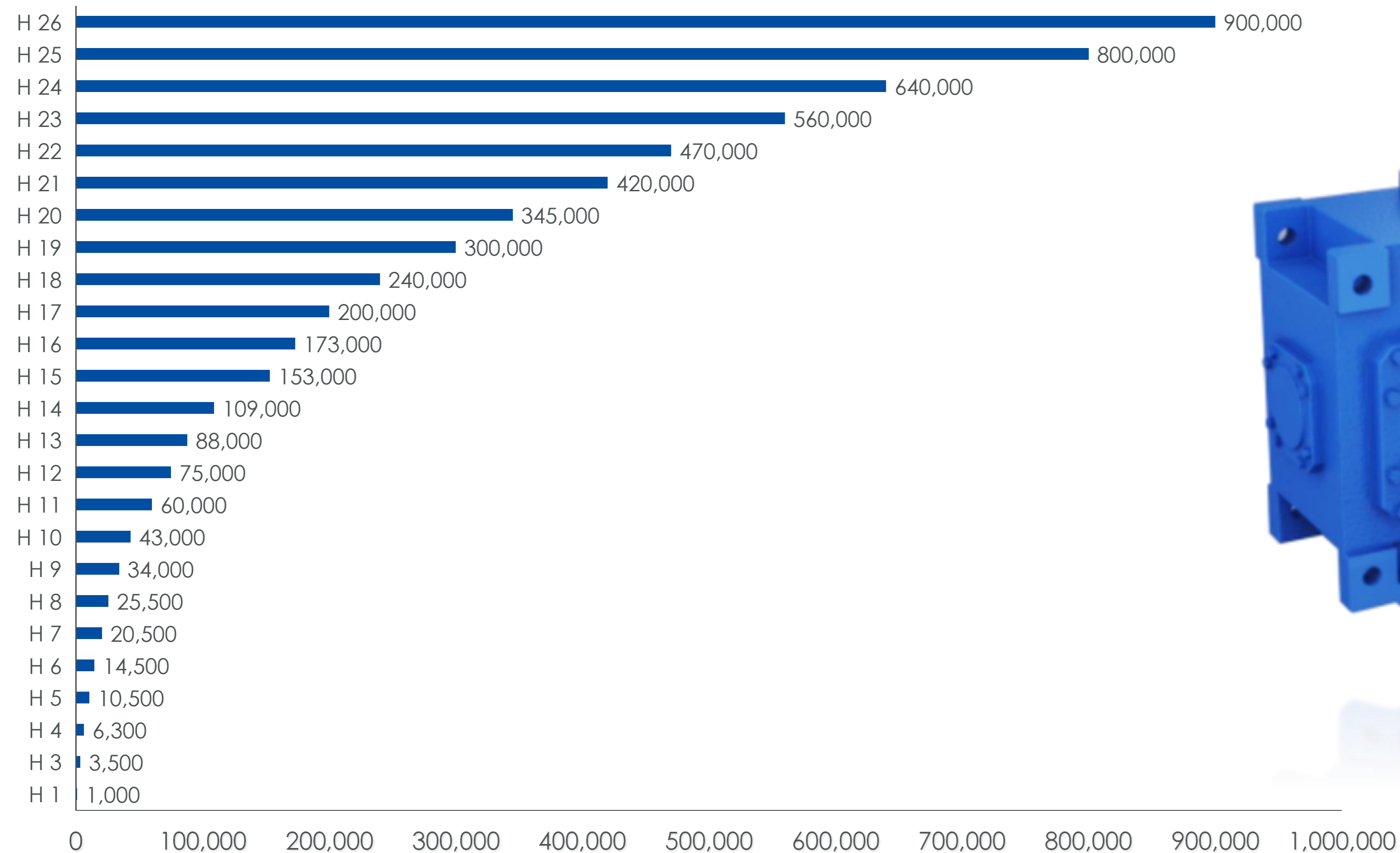
Maximum torque (N.m)
